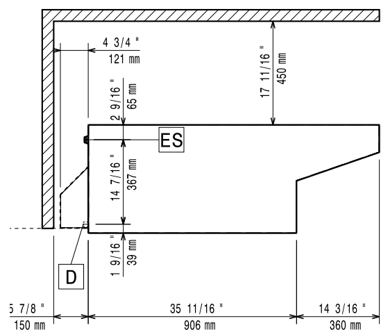
Oldalnézet
