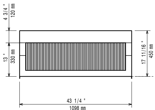
Oldalnézet
